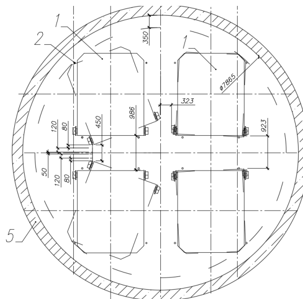
1 – подъемный сосуд (скуп СНМ 35-235-1,1); 2 – консольный расстрел; 3 – канатно-профильный проводник; 5 – крепь ствола.
