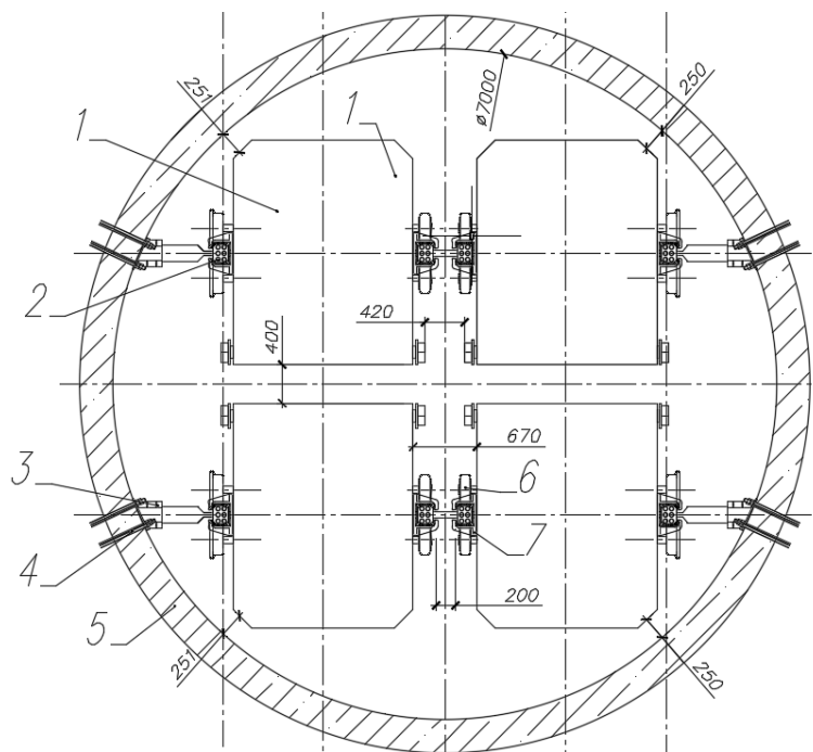
1 – подъемный сосуд (скап СНМ 35-235-1,1); 2 – КПП; 3 – консольный расстрел; 4 – анкера; 5 – крепь ствола; 6 – роликовые направляющие; 7 – предохранительная лапа
